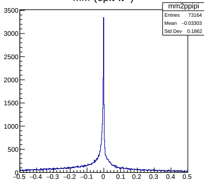
MM^2(e\pi\pi^+)
