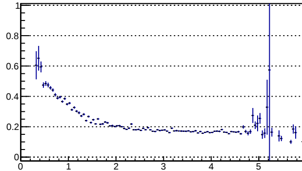
Fit Sigma V P
