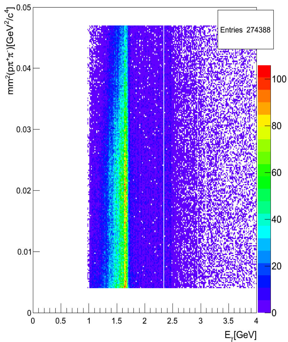
\text{mm}^2(\rho\pi^+\pi^-) VS E_\gamma
