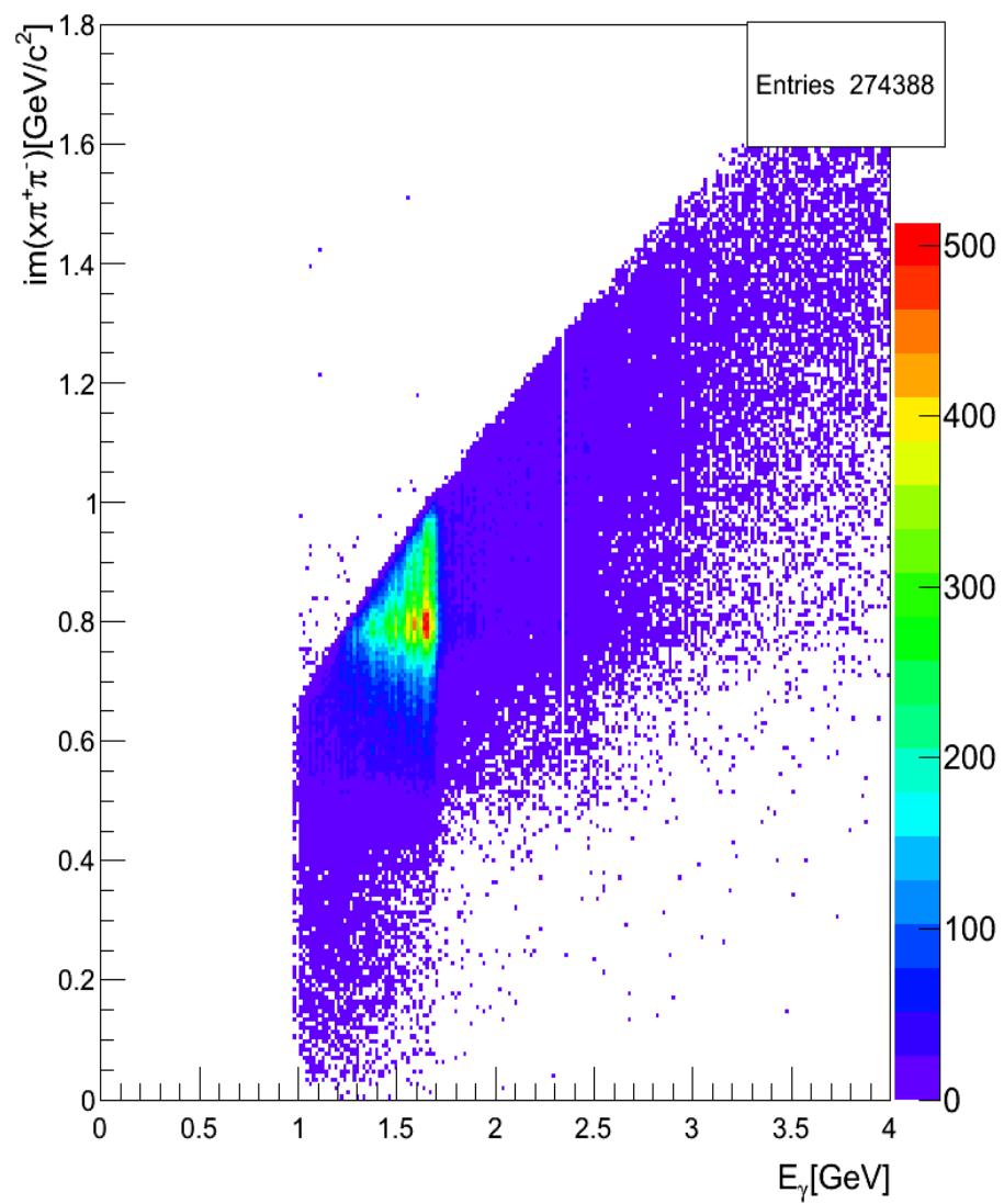
\text{im}(\chi\pi^+\pi^-) VS E_\gamma
