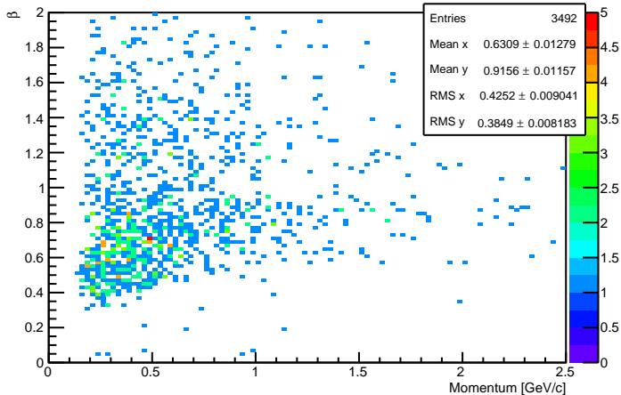
PID=9 (Pi-), dNumParticleVotes&gt;=2
