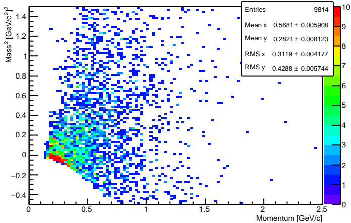
PID=8 (Pi+), dNumParticleVotes&gt;=2
