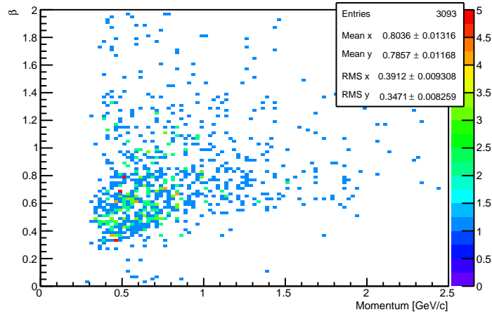
PID=14 (Proton), dNumParticleVotes&gt;=2
