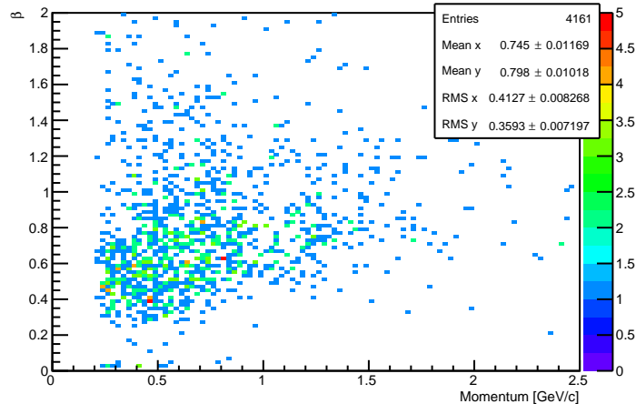
PID=11 (K+), dNumParticleVotes&gt;=2
