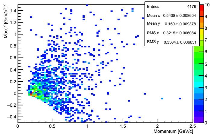
PID=9 (Pi-), dNumParticleVotes>=2
