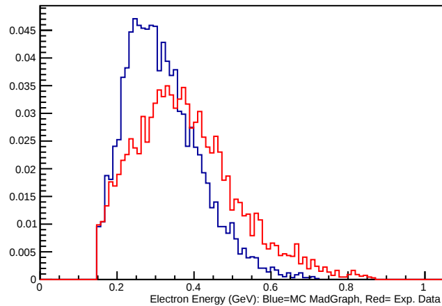
Em MadGraph
