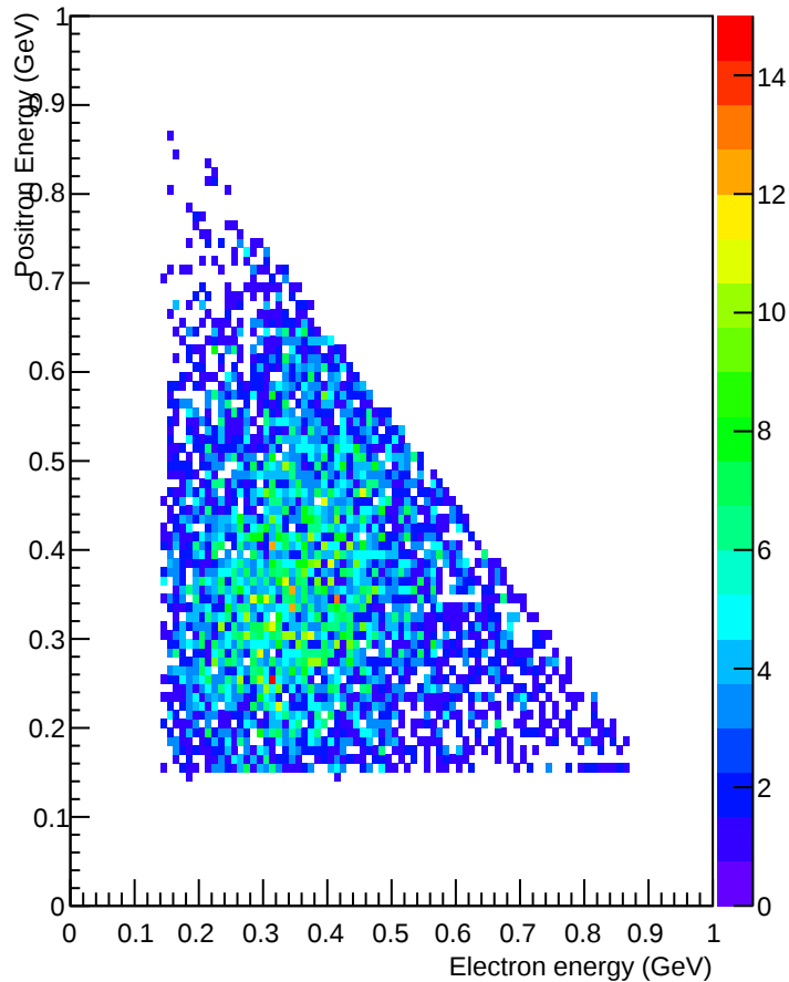
Ep VS Em Exp
