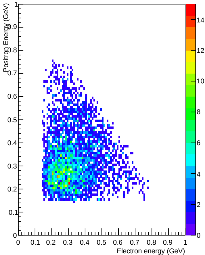
Ep VS Em VEGAS
