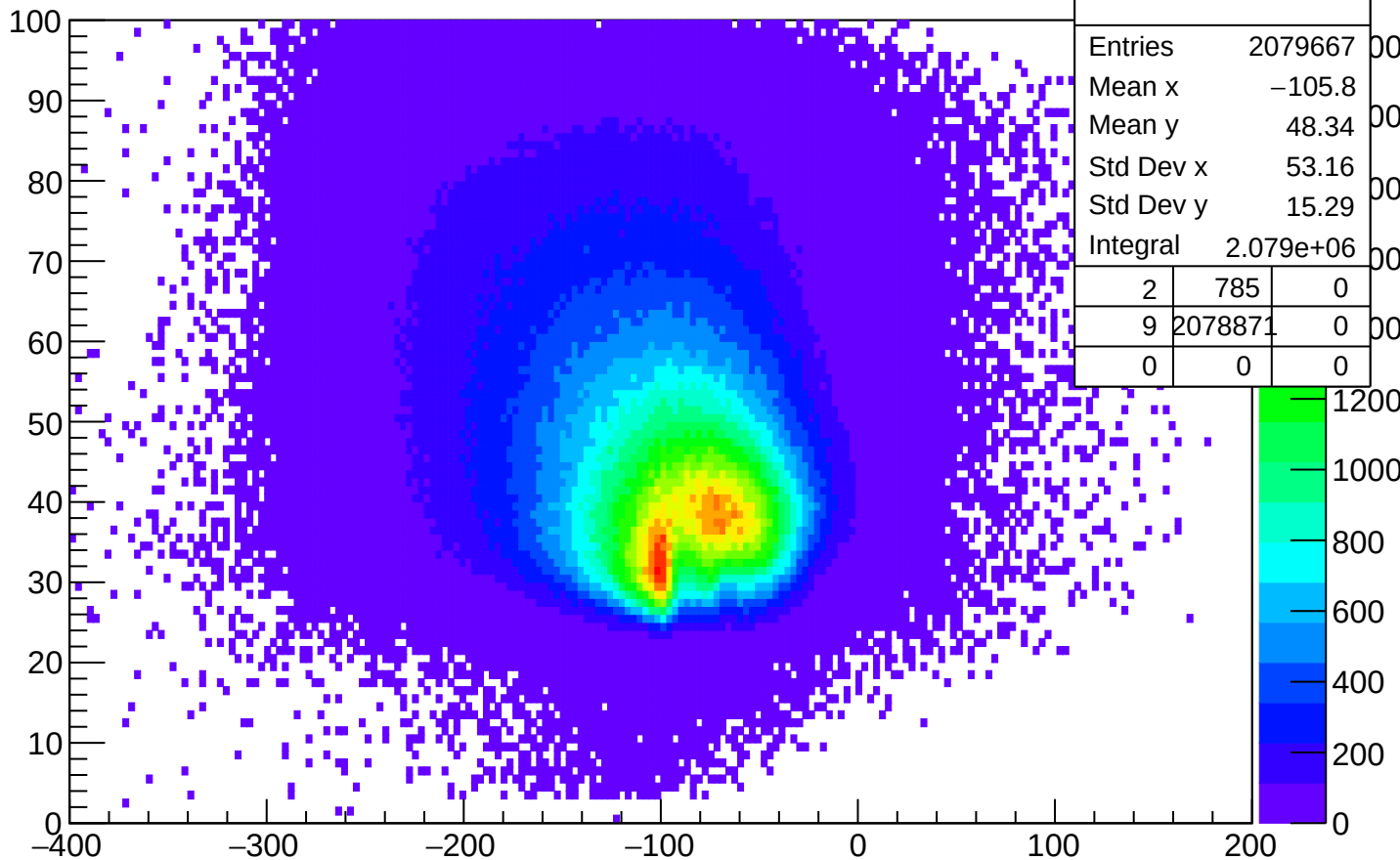
abs(eleTrkEcalY):eleTrkEcalX
