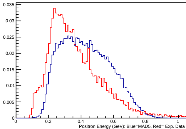
Positron Energy
