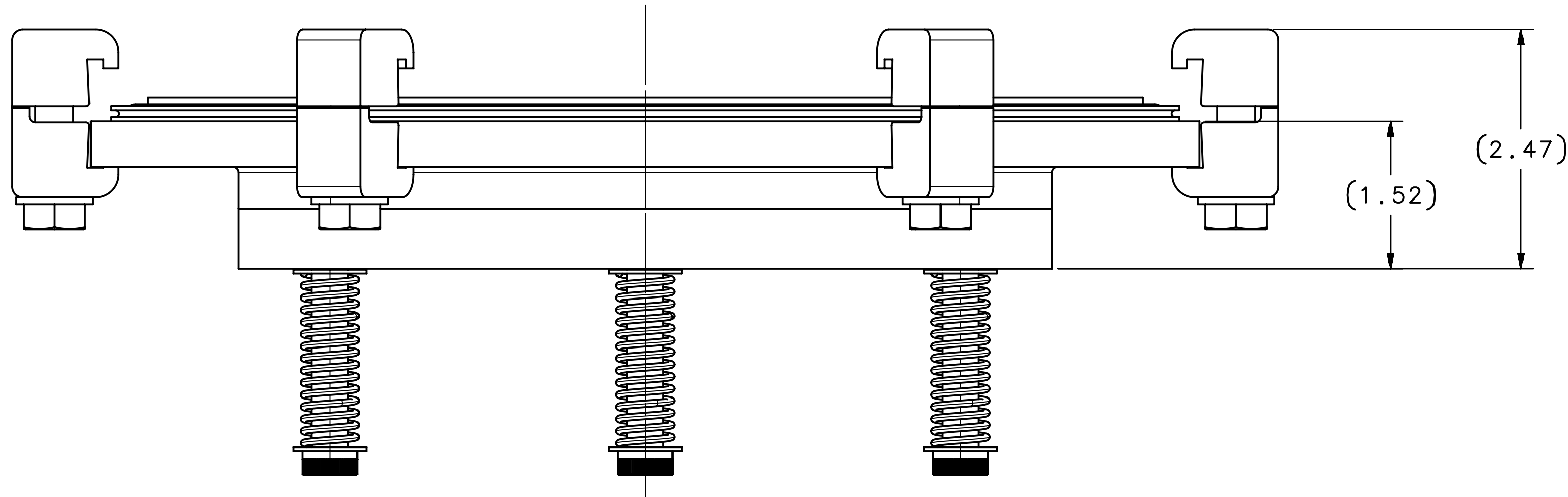
EDGE VIEW
