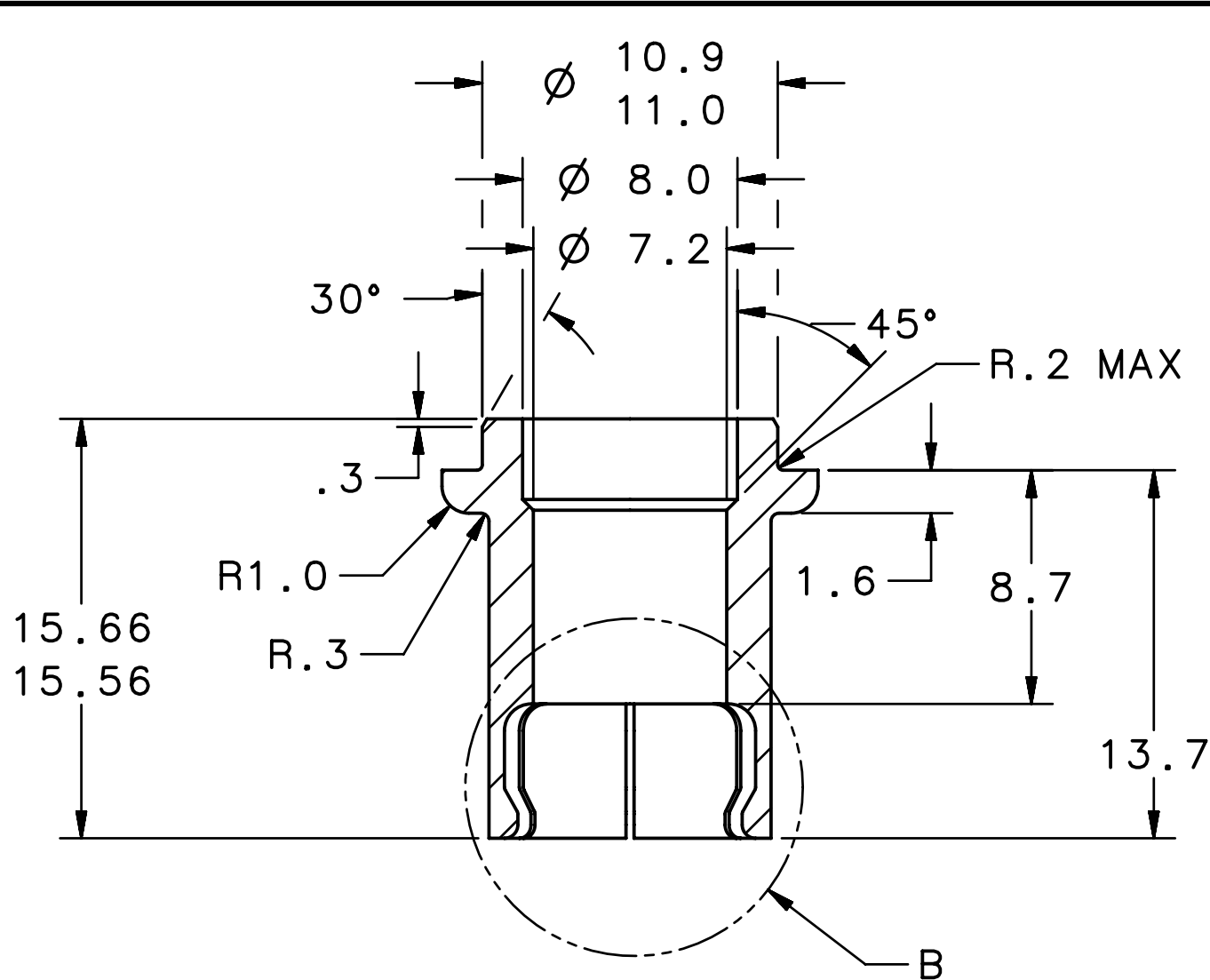
SECTION A-A
