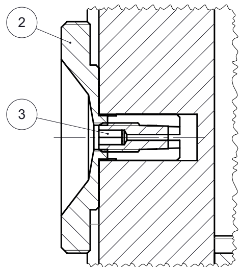
SEZIONE / SECTION A-A SCALA / SCALE 1.5:1
