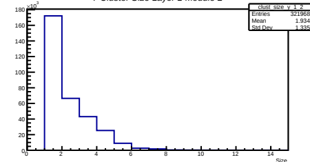
Y Cluster Size Layer 1 Module 2
