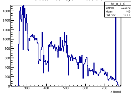
X Cluster Pos Layer 1 Module 0
