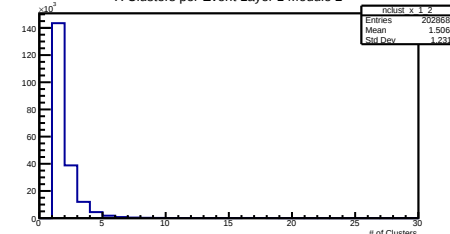
X Clusters per Event Layer 1 Module 2
