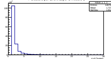
Y Clusters per Event Layer 1 Module 1
