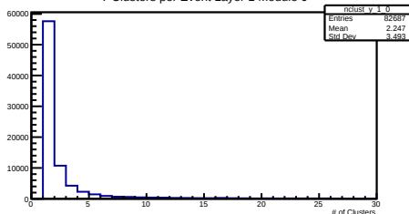
Y Clusters per Event Layer 1 Module 0
