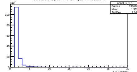
X Clusters per Event Layer 1 Module 1
