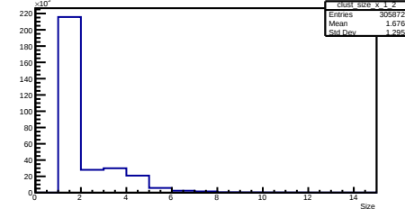
X Cluster Size Layer 1 Module 2
