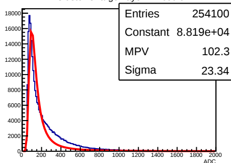
Y Cluster Charge Layer 1 Module 1
