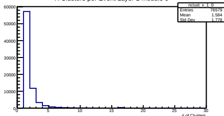
X Clusters per Event Layer 1 Module 0
