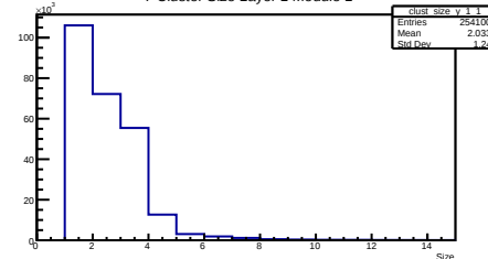
Y Cluster Size Layer 1 Module 1
