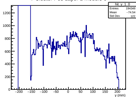
Y Cluster Pos Layer 1 Module 0
