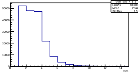
X Cluster Size Layer 1 Module 1
