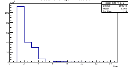
Y Cluster Size Layer 1 Module 0
