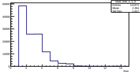
X Cluster Size Layer 1 Module 0
