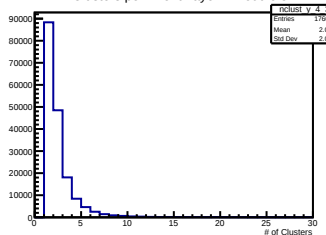
Y Clusters per Event Layer 4 Module 3
