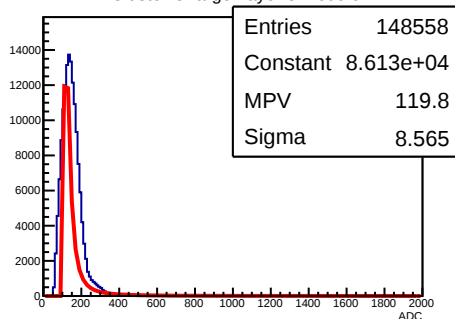
Y Cluster Charge Layer 3 Module 1
