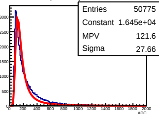
Y Strip ADC Layer 4 Module 3
