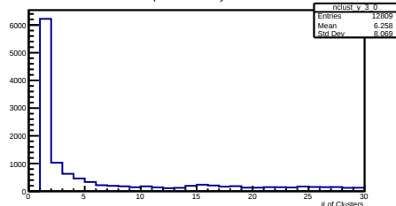
Y Clusters per Event Layer 3 Module 0
