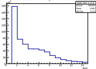
Y Cluster Size Layer 4 Module 0
