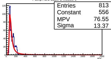
Y Strip ADC Layer 3 Module 0
