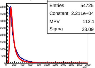
Y Strip ADC Layer 4 Module 2
