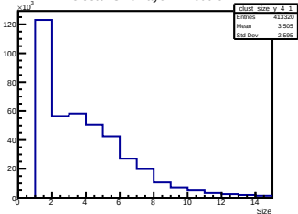
Y Cluster Size Layer 4 Module 1
