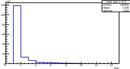
Y Cluster Size Layer 3 Module 1
