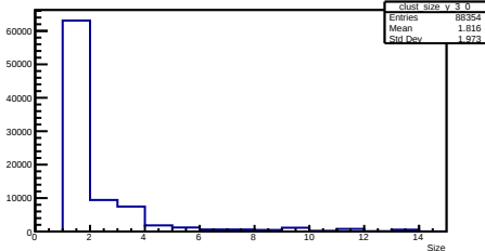
Y Cluster Size Layer 3 Module 0
