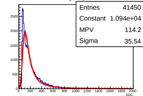
Y Cluster Charge Layer 1 Module 0
