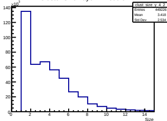
Y Cluster Size Layer 4 Module 2
