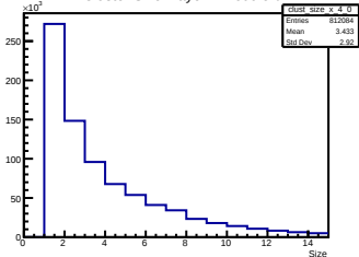
X Cluster Size Layer 4 Module 0
