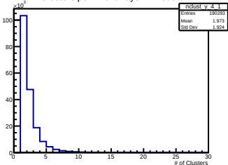
Y Clusters per Event Layer 4 Module 1
