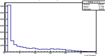
X Clusters per Event Layer 3 Module 1
