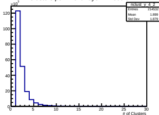
Y Clusters per Event Layer 4 Module 2
