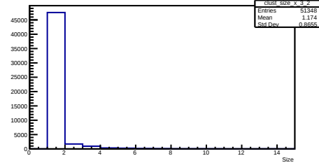
X Cluster Size Layer 3 Module 2
