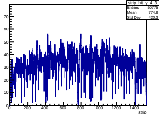
Y Strip Pos Layer 4 Module 3
