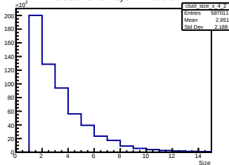
X Cluster Size Layer 4 Module 2
