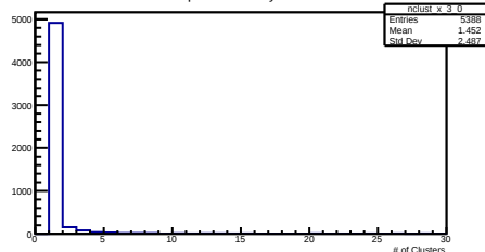
X Clusters per Event Layer 3 Module 0
