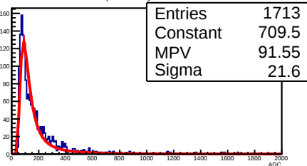
Y Strip ADC Layer 1 Module 0
