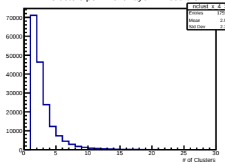
X Clusters per Event Layer 4 Module 3
