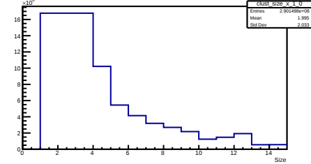
X Cluster Size Layer 1 Module 0
