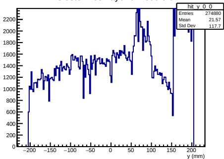
Y Cluster Pos Layer 0 Module 0
