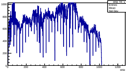
Y Strip Pos Layer 0 Module 0
