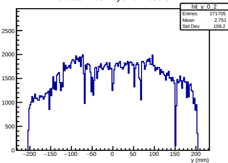
Y Cluster Pos Layer 0 Module 2
