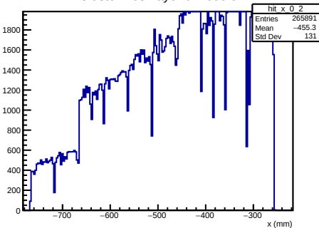
X Cluster Pos Layer 0 Module 2
