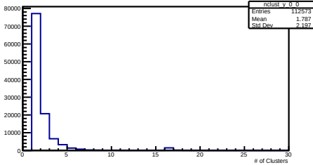
Y Clusters per Event Layer 0 Module 0
