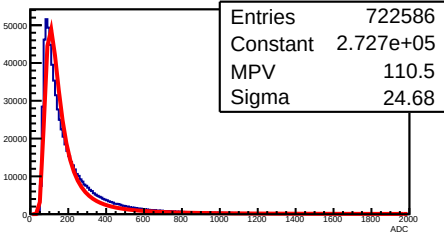
X Strip ADC Layer 0 Module 2
