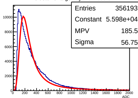
Y Cluster Charge Layer 0 Module 1
