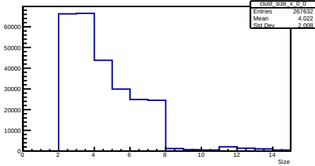
X Cluster Size Layer 0 Module 0
