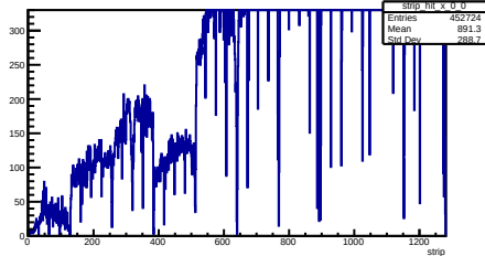
X Strip Pos Layer 0 Module 0
