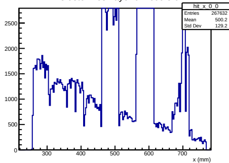
X Cluster Pos Layer 0 Module 0
