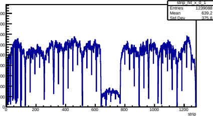
X Strip Pos Layer 0 Module 1
