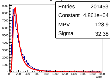
Y Cluster Charge Layer 0 Module 0
