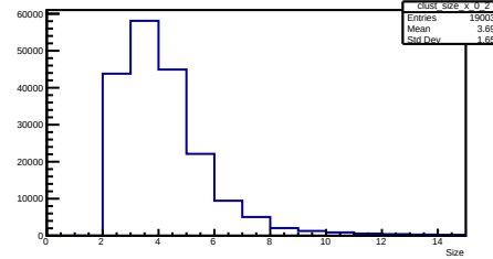
X Cluster Size Layer 0 Module 2
