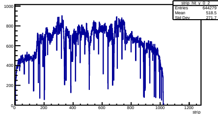
Y Strip Pos Layer 0 Module 2
