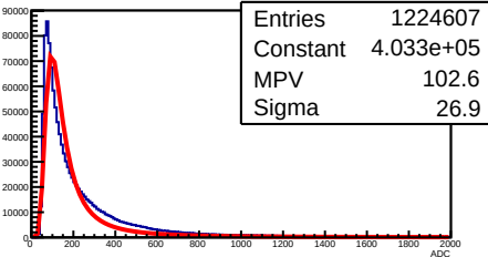
Y Strip ADC Layer 0 Module 1
