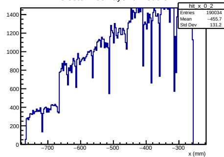
X Cluster Pos Layer 0 Module 2
