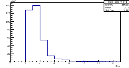
Y Cluster Size Layer 0 Module 1
