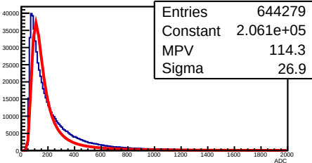
Y Strip ADC Layer 0 Module 2
