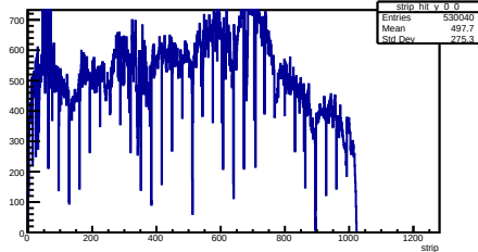
Y Strip Pos Layer 0 Module 0
