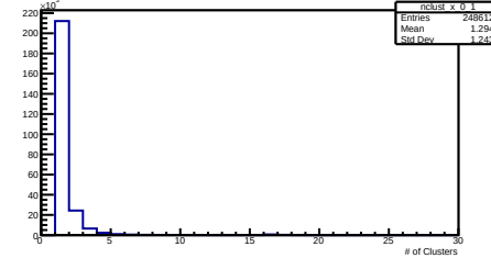
X Clusters per Event Layer 0 Module 1
