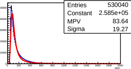
Y Strip ADC Layer 0 Module 0
