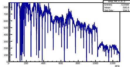
X Strip Pos Layer 0 Module 2
