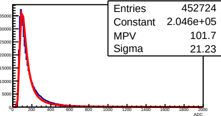
X Strip ADC Layer 0 Module 0
