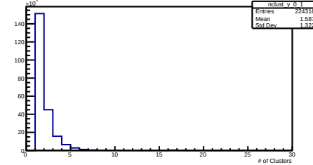
Y Clusters per Event Layer 0 Module 1
