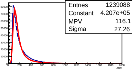
X Strip ADC Layer 0 Module 1
