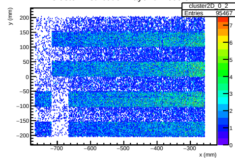
Cluster Distribution Layer 0 Module 2
