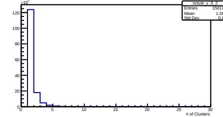
Y Clusters per Event Layer 0 Module 2
