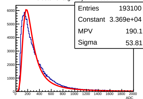
Y Cluster Charge Layer 0 Module 2
