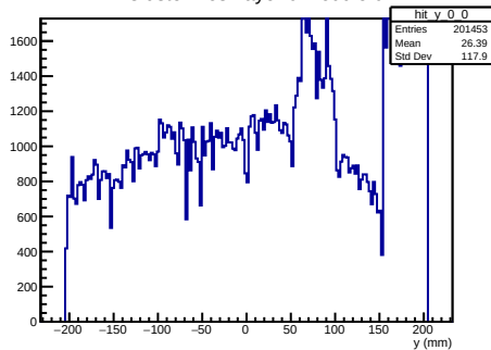
Y Cluster Pos Layer 0 Module 0
