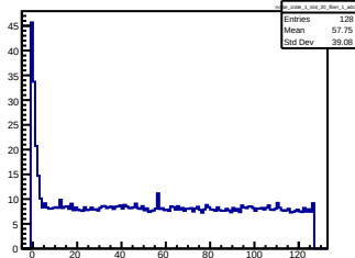
noise_crate_1_slot_20_fiber_1_adc_5
