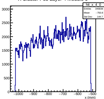
X Cluster Pos Layer 4 Module 0
