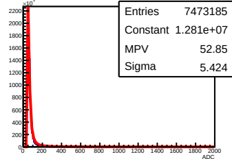
Y Strip ADC Layer 4 Module 3
