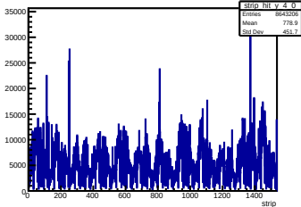
Y Strip Pos Layer 4 Module 0
