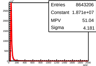
Y Strip ADC Layer 4 Module 0
