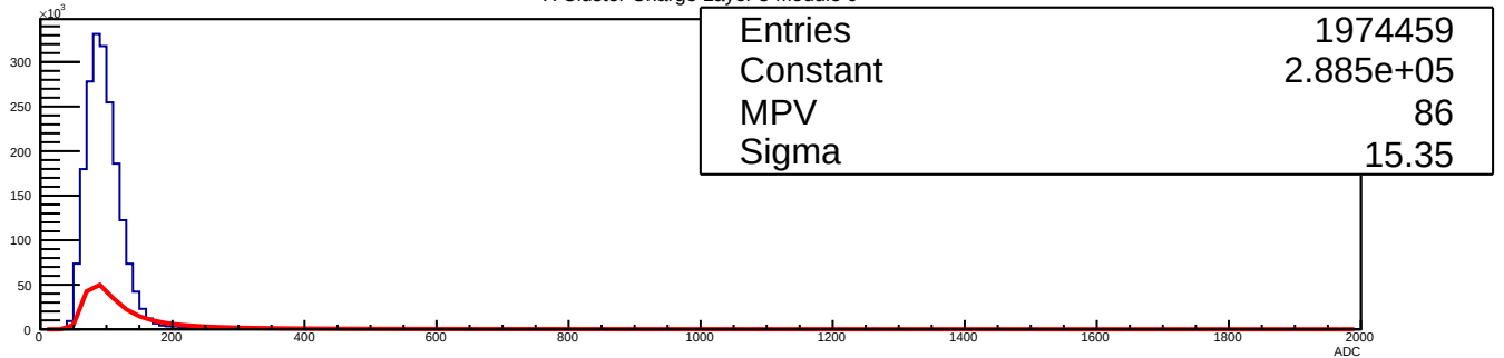
Y Cluster Charge Layer 3 Module 0
