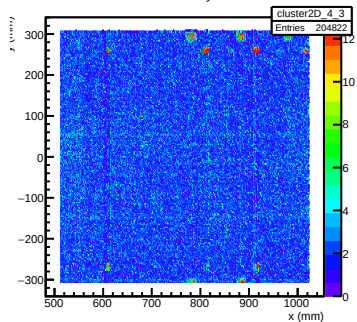
Cluster Distribution Layer 4 Module 3
