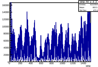
Y Strip Pos Layer 4 Module 2
