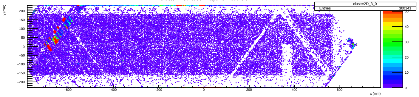
X Cluster Pos Layer 3 Module 0
