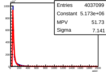
X Strip ADC Layer 4 Module 2
