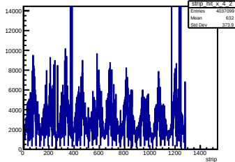
X Strip Pos Layer 4 Module 2
