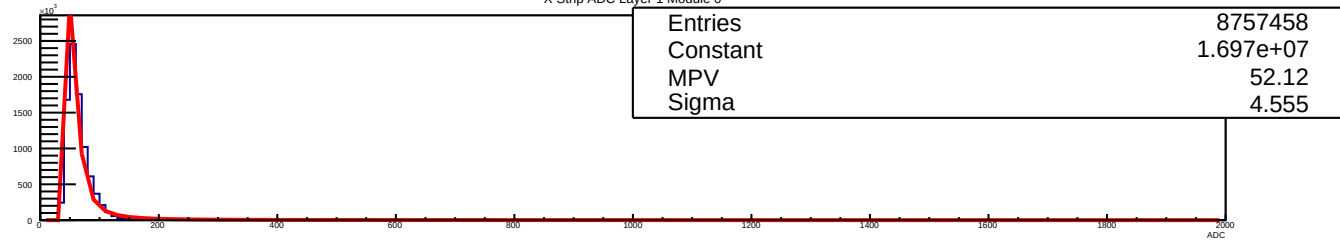
Y Strip ADC Layer 1 Module 0
