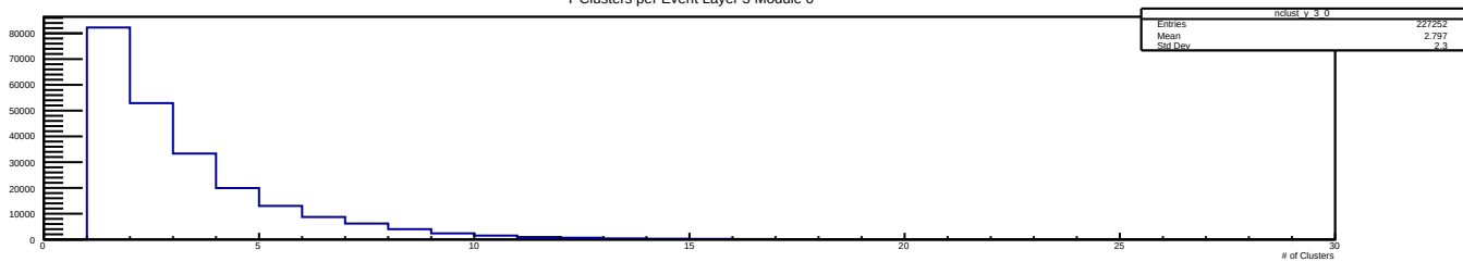
Y Clusters per Event Layer 3 Module 0
