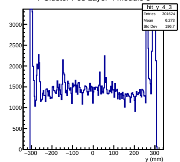
Y Cluster Pos Layer 4 Module 3
