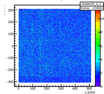
Cluster Distribution Layer 4 Module 2
