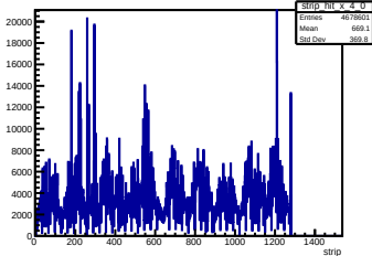
X Strip Pos Layer 4 Module 0
