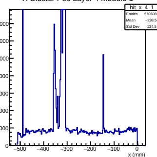
X Cluster Pos Layer 4 Module 1
