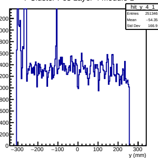
Y Cluster Pos Layer 4 Module 1
