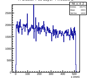
X Cluster Pos Layer 4 Module 2
