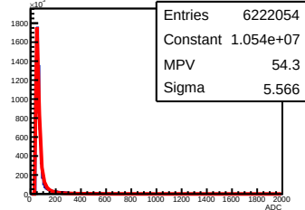
Y Strip ADC Layer 4 Module 2
