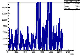
X Strip Pos Layer 4 Module 3
