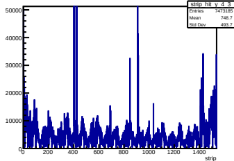
Y Strip Pos Layer 4 Module 3
