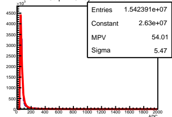
Y Strip ADC Layer 4 Module 2
