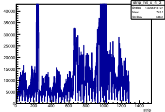
X Strip Pos Layer 4 Module 3
