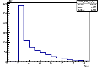
X Cluster Size Layer 4 Module 1
