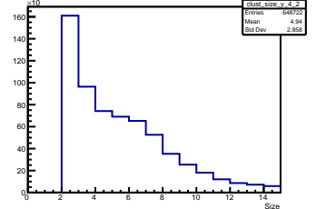
Y Cluster Size Layer 4 Module 2
