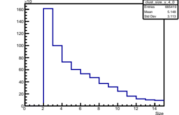
Y Cluster Size Layer 4 Module 0
