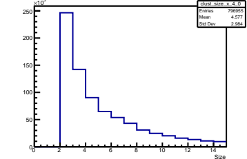
X Cluster Size Layer 4 Module 0
