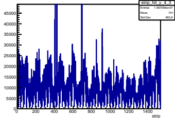
Y Strip Pos Layer 4 Module 3
