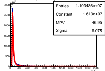
X Strip ADC Layer 4 Module 0
