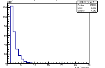
Y Clusters per Event Layer 4 Module 1
