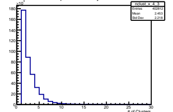
X Clusters per Event Layer 4 Module 3
