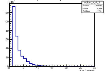
X Clusters per Event Layer 4 Module 2
