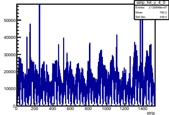
Y Strip Pos Layer 4 Module 0
