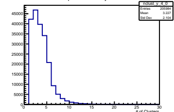
Y Clusters per Event Layer 4 Module 0
