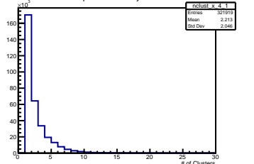
X Clusters per Event Layer 4 Module 1
