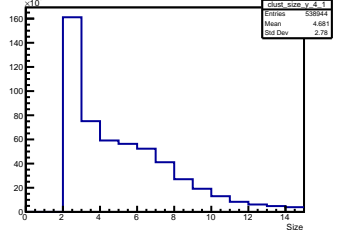
Y Cluster Size Layer 4 Module 1
