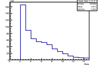
Y Cluster Size Layer 4 Module 3
