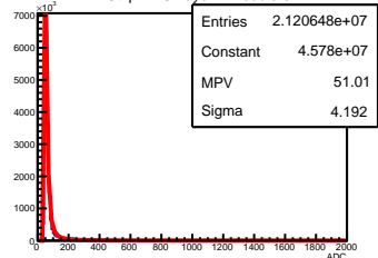
Y Strip ADC Layer 4 Module 0
