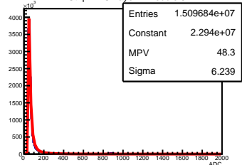
X Strip ADC Layer 4 Module 3
