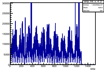
X Strip Pos Layer 4 Module 2
