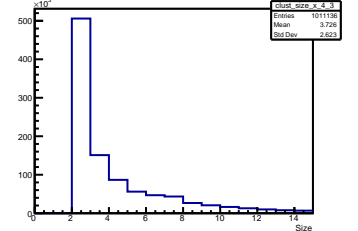
X Cluster Size Layer 4 Module 3
