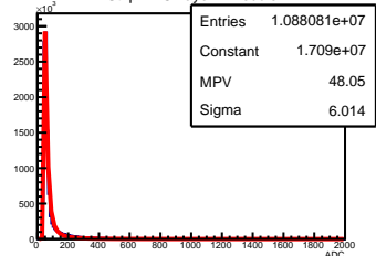
X Strip ADC Layer 4 Module 1
