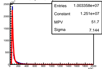
X Strip ADC Layer 4 Module 2
