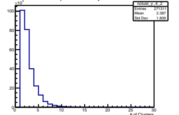
Y Clusters per Event Layer 4 Module 2
