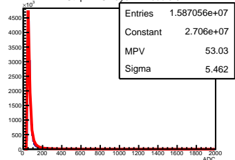
Y Strip ADC Layer 4 Module 3
