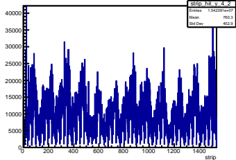
Y Strip Pos Layer 4 Module 2
