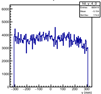
Y Cluster Pos Layer 4 Module 0
