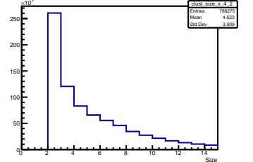
X Cluster Size Layer 4 Module 2
