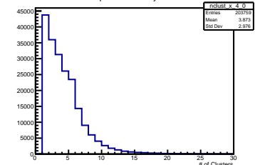
X Clusters per Event Layer 4 Module 0
