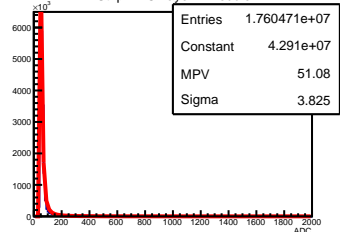
Y Strip ADC Layer 4 Module 1
