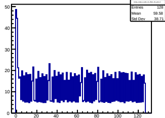
noise_crate_4_slot_11_fiber_16_adc_0
